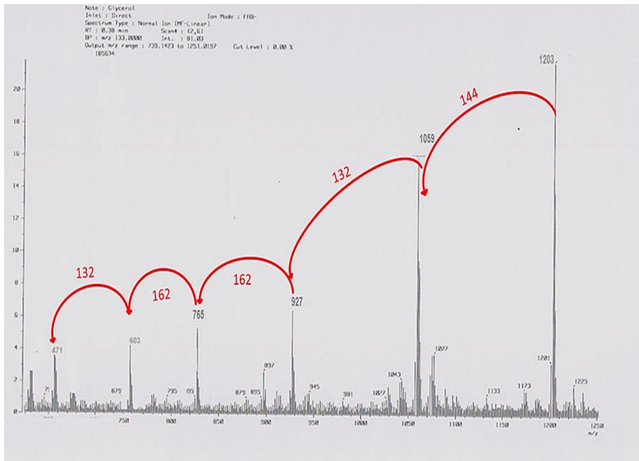
Figure N°62 : Spectre de masse en source FAB (en mode négatif) composé 5
