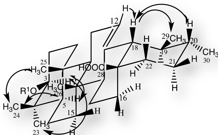
Fig. 75 Steréochimie de l'aglycone du composé 1 , NOESY correlations
