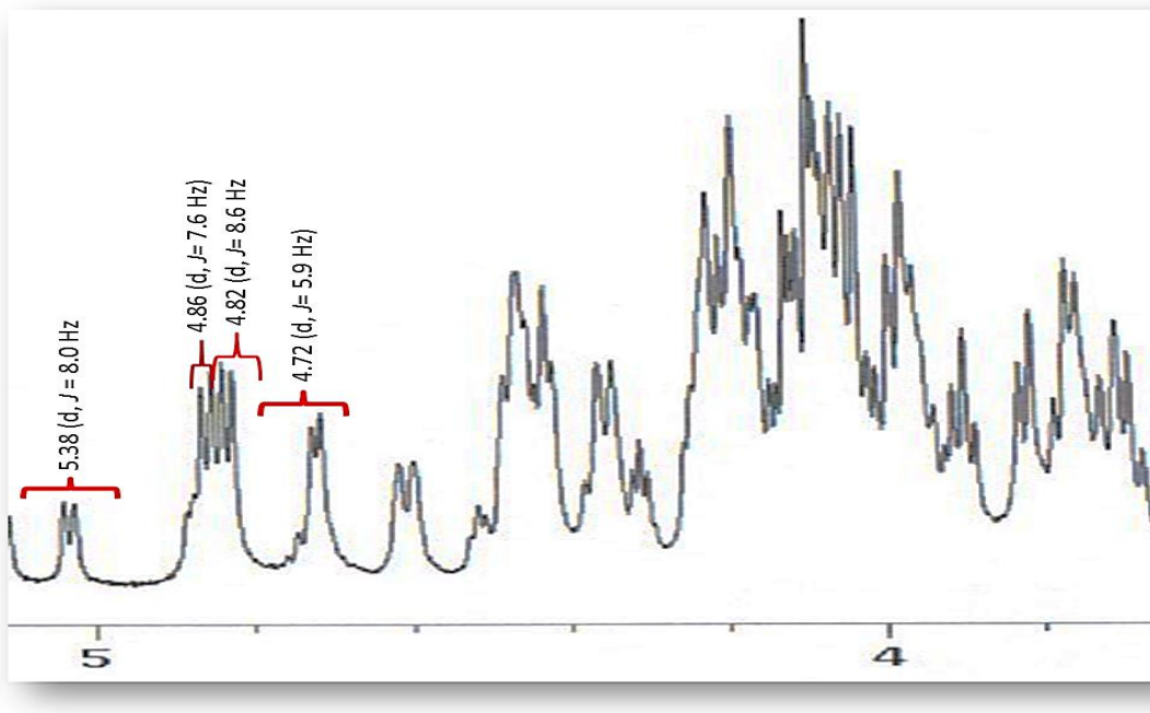
Figure N° 40 : Spectre RMN 1 H des protons anomériques du composé 1.
