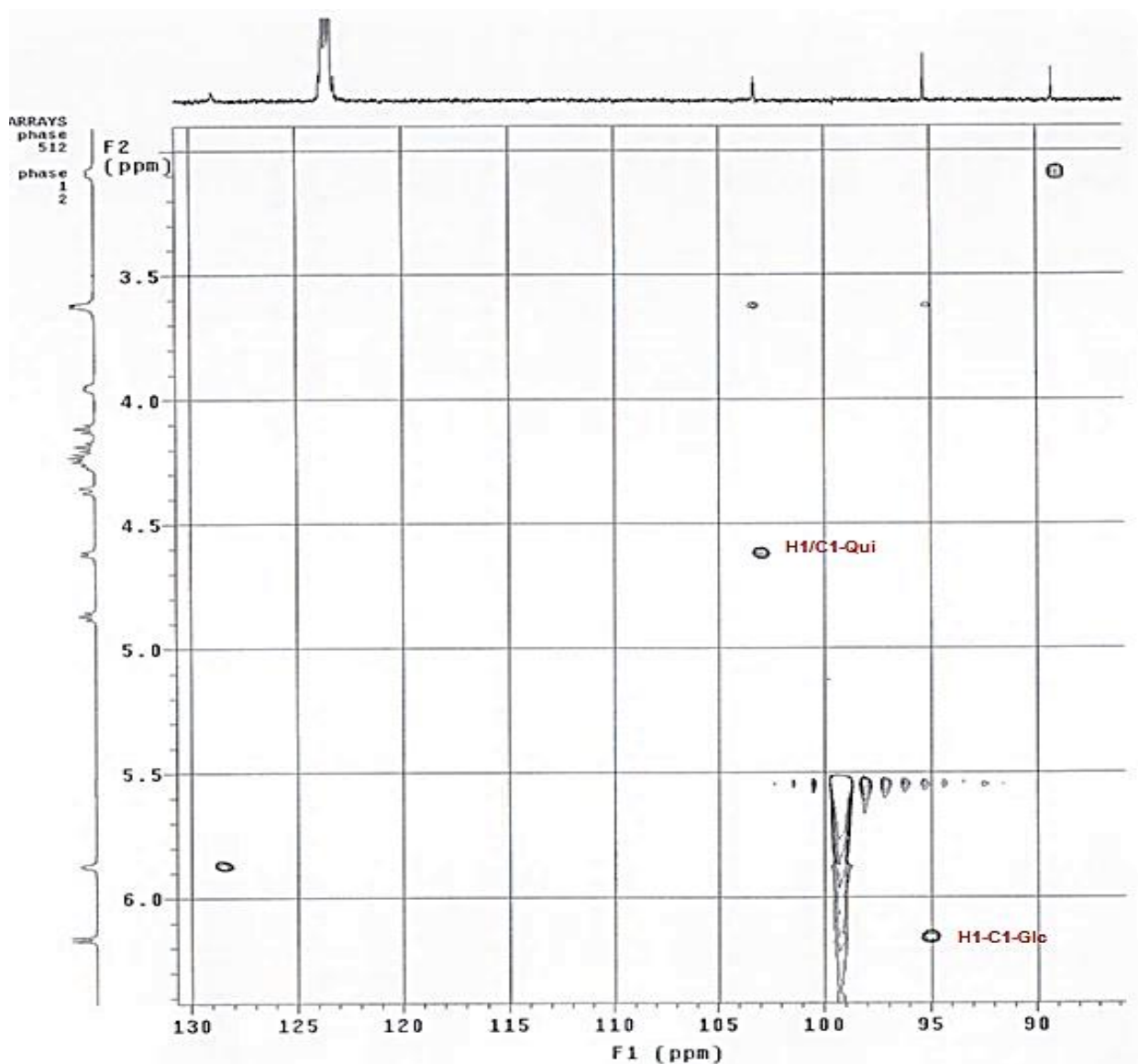
Figure N°92: Spectre HSQC du composé 5 (zone des anomères)
