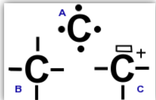
Figure N°15: Formule de Lewis.
